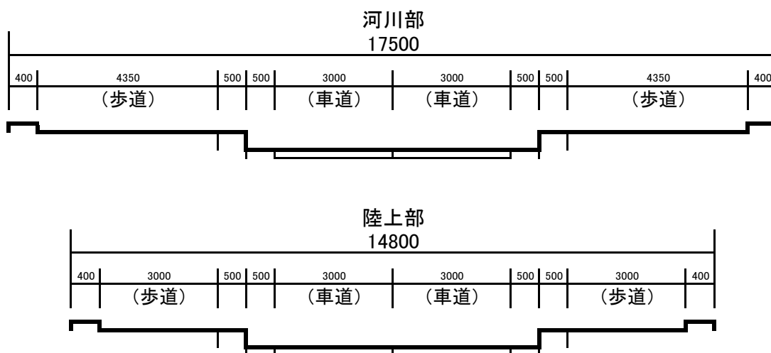
【標準横断面図】
