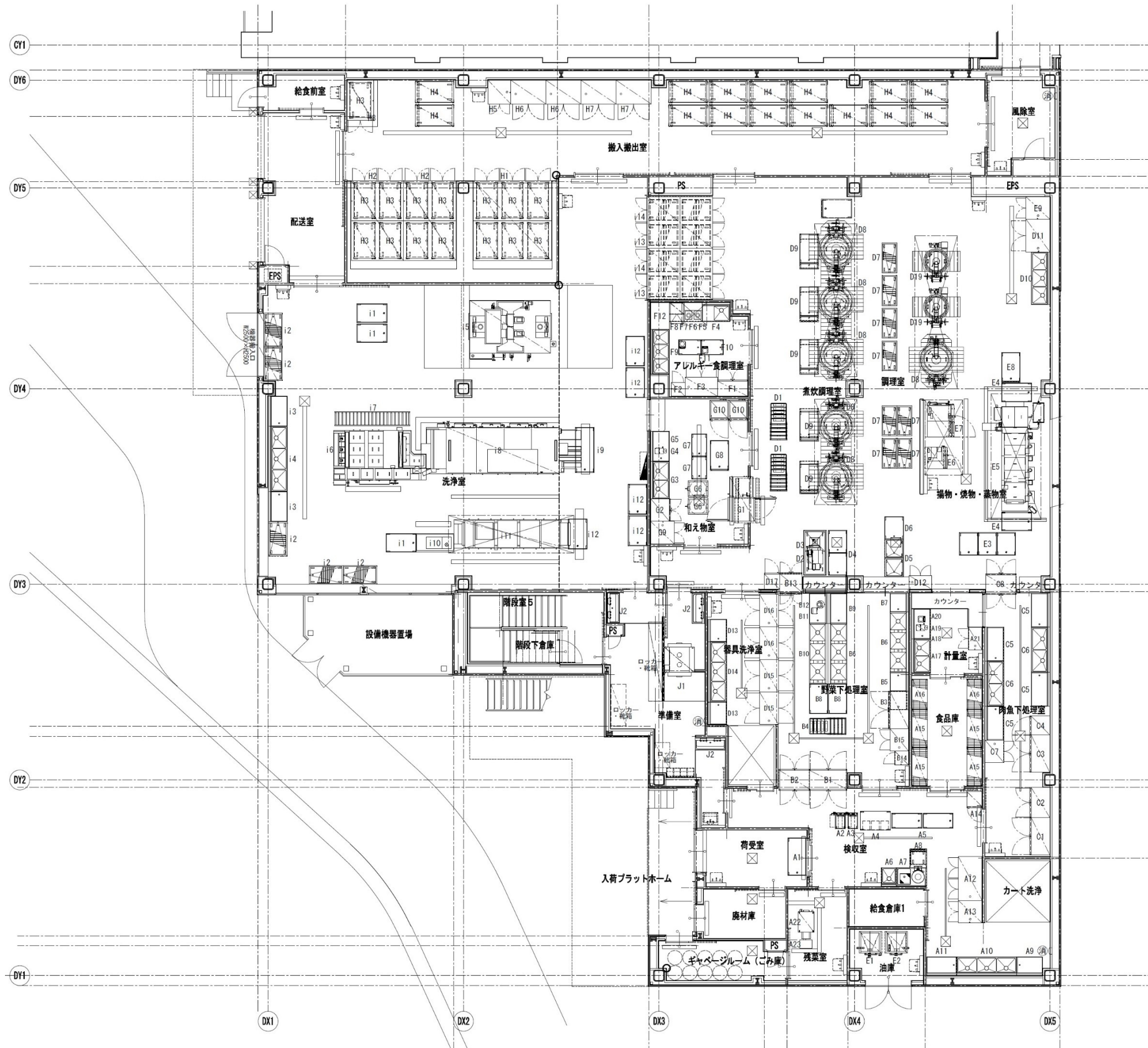
別紙2-① 1階施設平面図(機器番号入)
